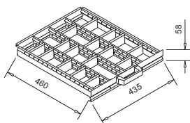
GAVETA PEQUENA Divisórias Removíveis Vãos a partir de 90x25mm
