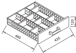
GAVETA MÉDIA Divisórias Removíveis Vãos a partir de 130x25mm
