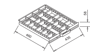
GAVETA PEQUENA Divisórias Removíveis Vãos a partir de 90X25mm
