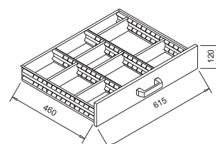
GAVETA MÉDIA Divisórias Removíveis Vãos a partir de 190x25mm
